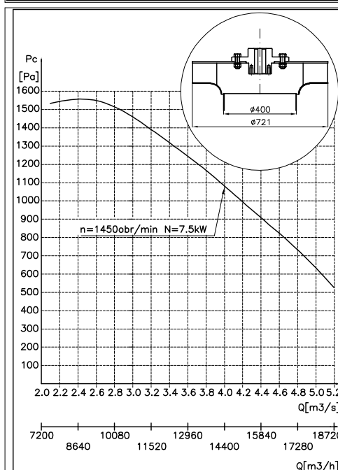
Charakterystyka teoret. WP400/721 napęd bezpośredni
