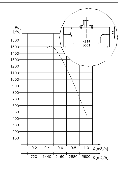
Charakterystyka teoret. WP219/351
