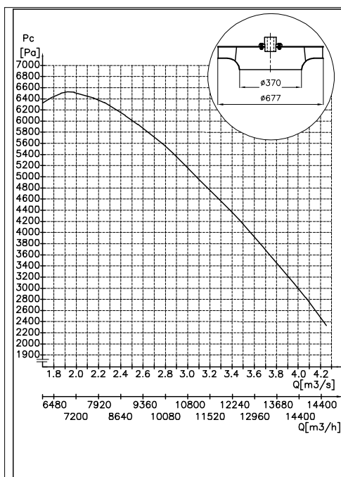
Charakterystyka teoret. WP355/677
