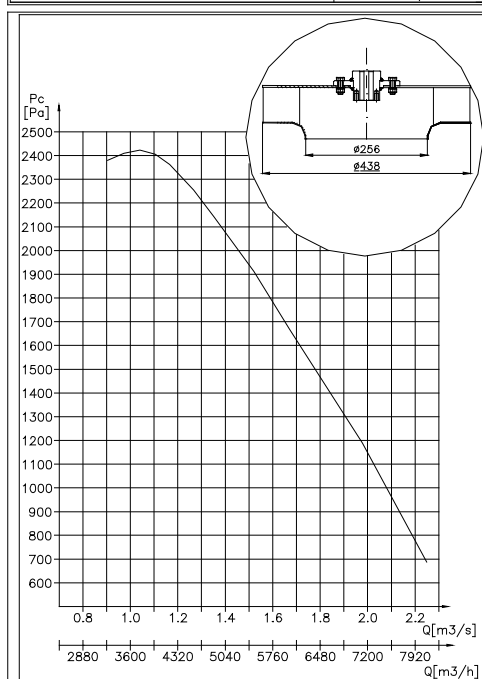
Charakterystyka teoret. WP256/438
