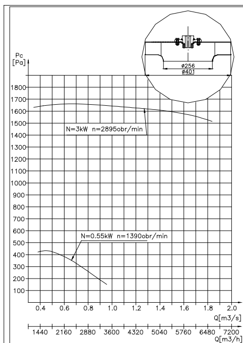
Charakterystyka teoret. WP256/401
