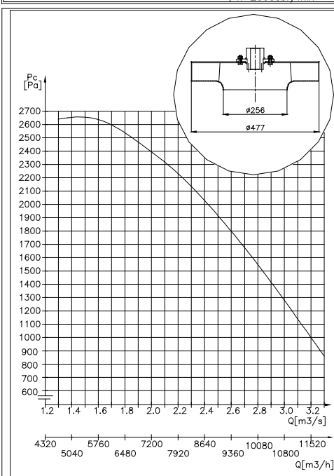
Charakterystyka teoret. WP256/477
