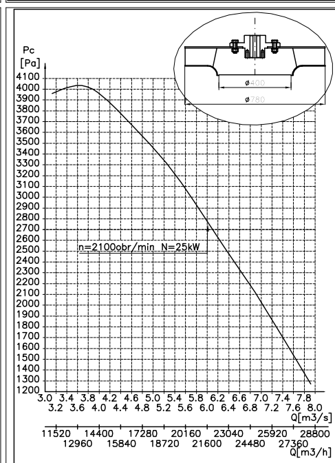
Charakterystyka teoret. WP400/780 napęd pasowy
