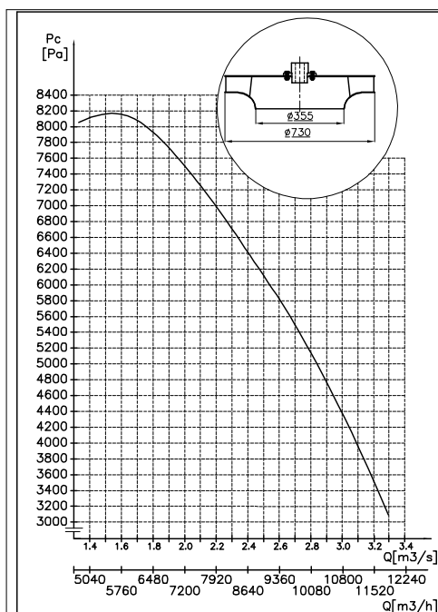
Charakterystyka teoret. WP355/730
