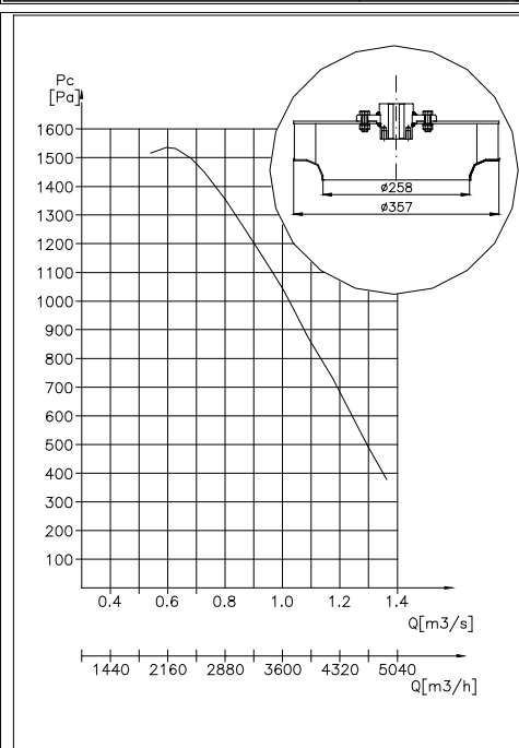
Charakterystyka teoret. WP256/357
