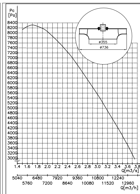
Charakterystyka teoret. WP355/736
