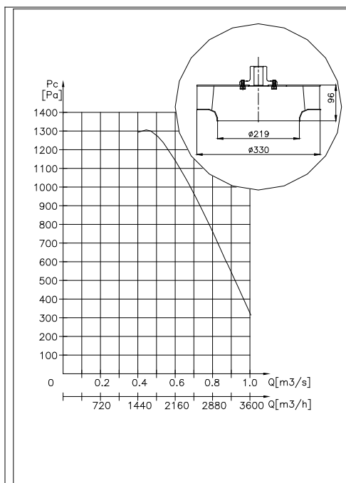
Charakterystyka teoret. WP219/330
