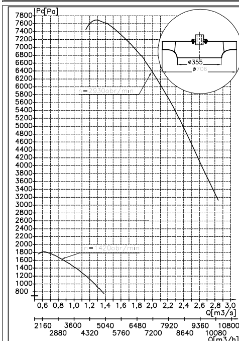
Charakterystyka teoret. WP355/706
