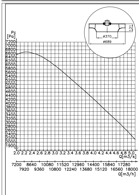
Charakterystyka teoret. WP355/689
