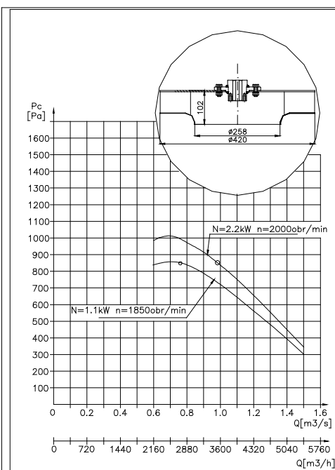
Charakterystyka teoret. WP256/420
