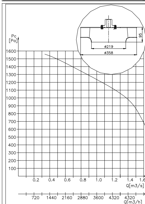
Charakterystyka teoret. WP219/358
