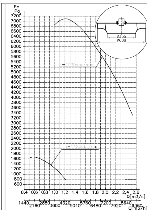
Charakterystyka teoret. WP355/688
