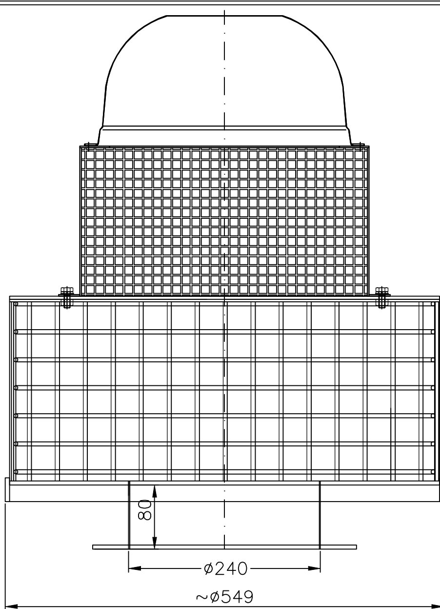
Kołnierz wlotu
